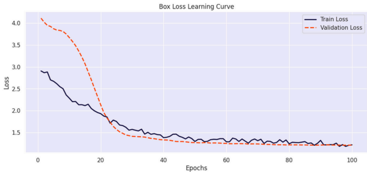
Hình 6. Box Loss mô hình YOLO.
