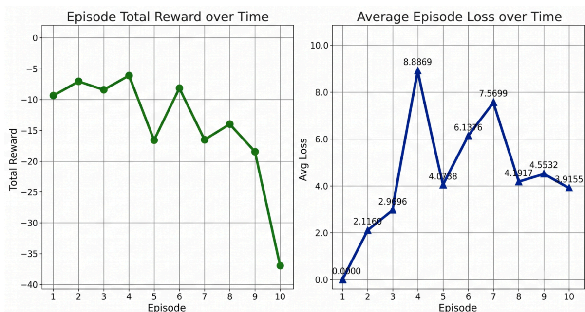
Hình 11 Hàm nhận phần thưởng và mất mát đánh giá độ hiệu quả của agent.
