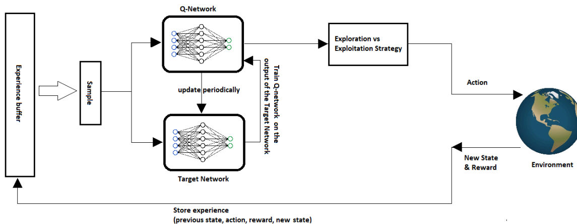
Hình 10. Mô hình DQN
