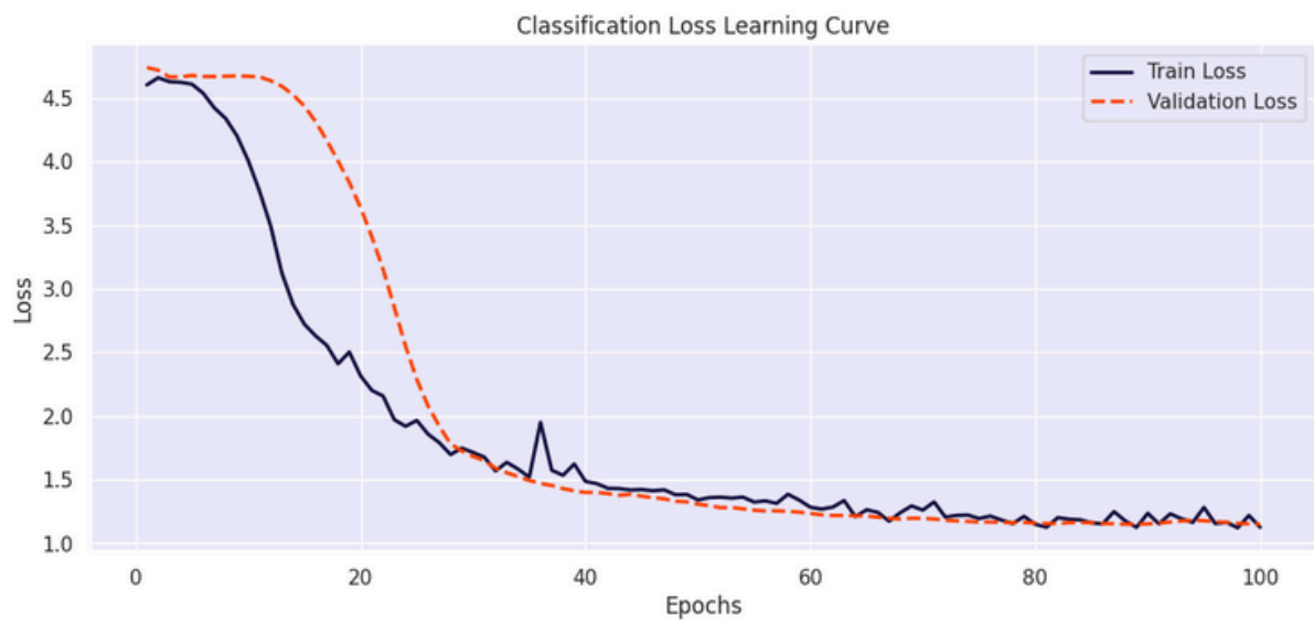
Hình 7. Classification Loss mô hình YOLO.
