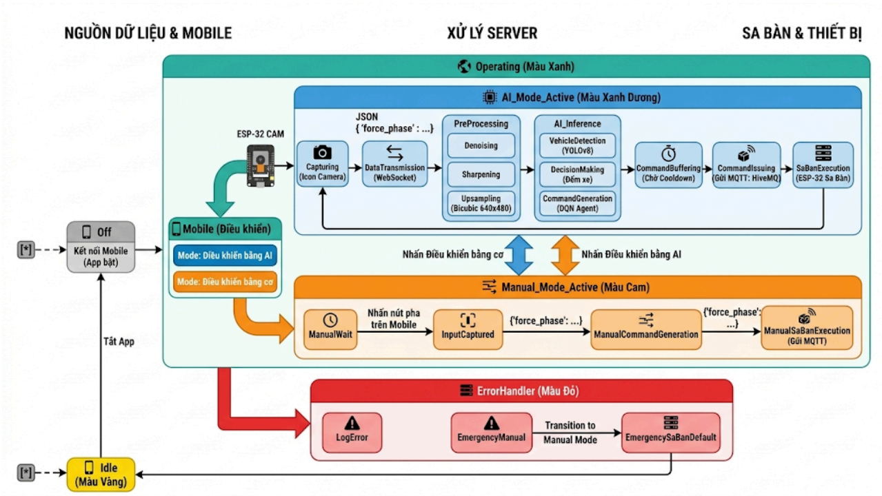
Hình 2. Luồng dữ liệu của hệ thống.
